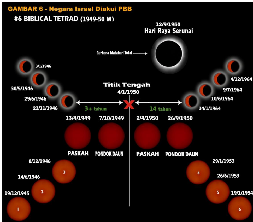
Gambar 6: Biblical Blood Moon Tetrad tahun 1949-1950. Terdapat 3 gerhana bulan total sebelum Biblical Blood Moon Tetrad dan 3 gerhana bulan total setelahnya. Terjadi juga 4 gerhana matahari
