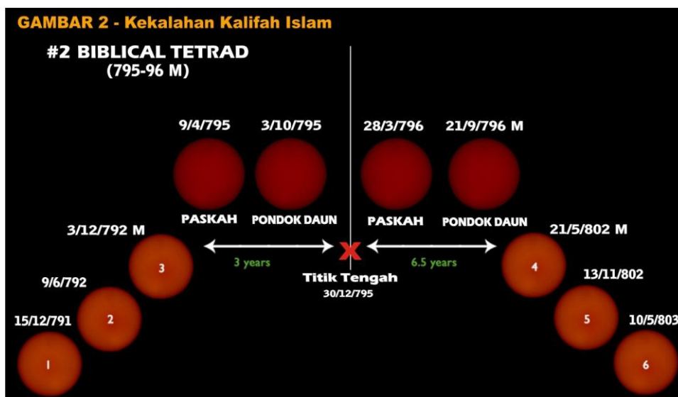
Gambar 2: Biblical Blood Moon Tetrad tahun 795□796 M. Terjadi 3 gerhana bulan total sebelum Biblical Blood Moon Tetrad dan 3 gerhana bulan total setelahnya.
